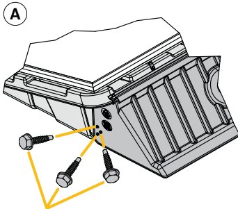
Sechskantbohrschrauben
